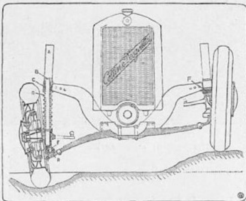
Новый способ подвески колес. „Независимые“ колеса системы „Cottin Desgouttes“. Общей оси нет. А — трубка, в которой скользит другая—ось колеса (В). С — предохранитель, не позволяющий трубке В выскакивать. D — гармоника из кожи, защищающая трубку В от грязи. E — тормоз на колеса. R — рессора
